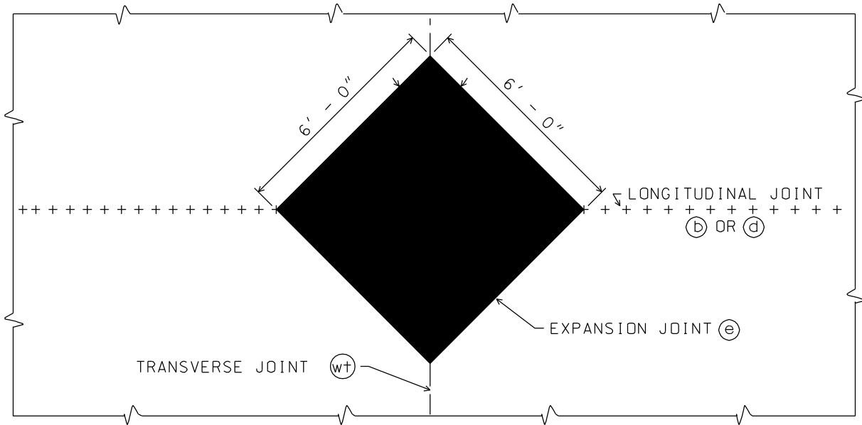
MANHOLE BOXOUT
